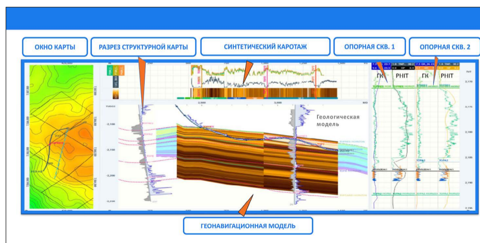
Процесс геонавигации горизонтальной скважины.
