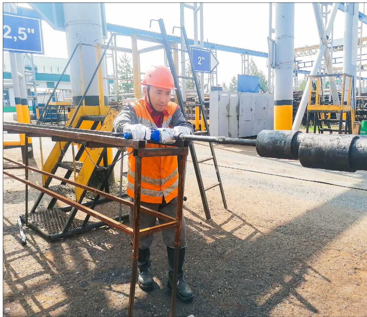
Установка для очистки труб, изготовленная силами ЦПО, испытывается на стенде. / ФОТО: РОБЕРТ БИЛАЛОВ, «ЕВС».
