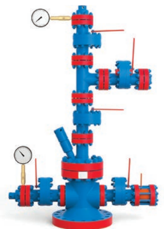
АФК1(Ш)-65x21K1(K2)M4 Базовый вариант
