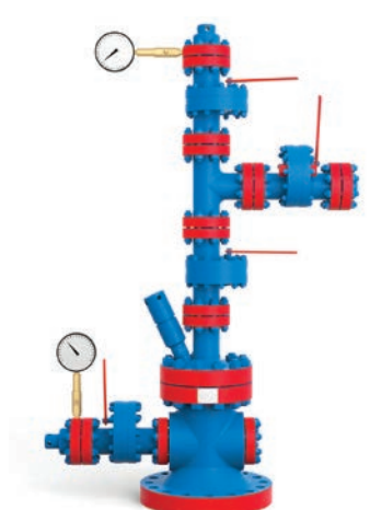
АФК1(Ш)-65x21K1(K2)M4-03 Без задвижки на боковом отводе крестовины
