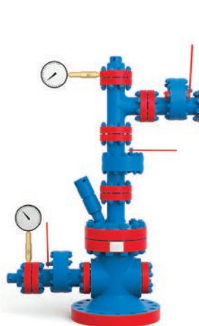
АФК1(Ш)-65x21K1(K2)M4-05 Без лубрикаторной задвижки и задвижки на боковом отводе крестовины
